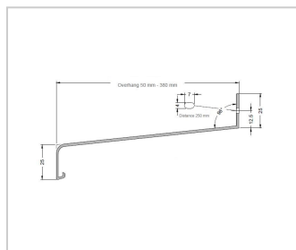
# 36. GUT GS 25/165 alumiiniumist veelaud 165mm BLANK 1pk=36m
