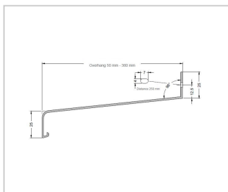
# 35. GUT GS 25/150 alumiiniumist veelaud 150mm BLANK 1pk=36m
